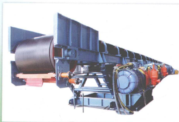
DSJ100/100/2×200 大功率长距离可伸缩皮带机
