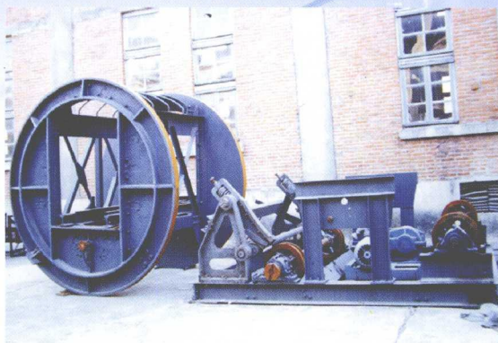
1 吨单车翻车机
