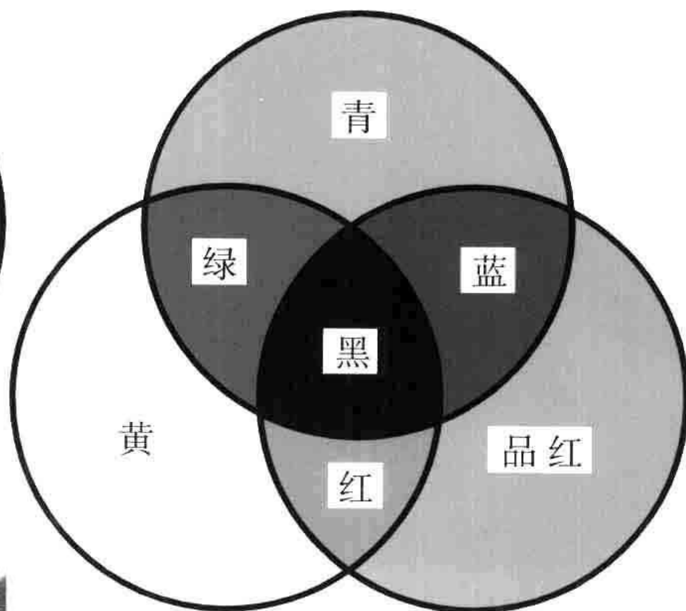
彩图 27-2 减色法色彩合成
