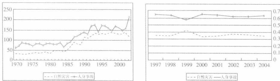
图 1-1 1970 年起全球自然灾害与人为事故发生数量与发生比例 ②
