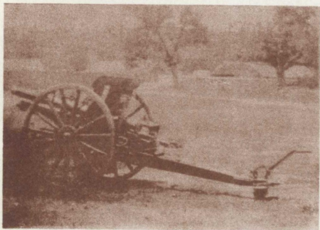
东三省兵工厂造民13式75（7.5 厘米）野炮（仿日本明治38年式）
