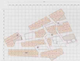
▲ 本层建筑面积 7900 m 2 街式商铺二层平面图
