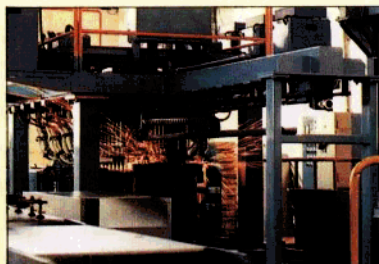
辊轧成形线上的箱体多头自动焊接
