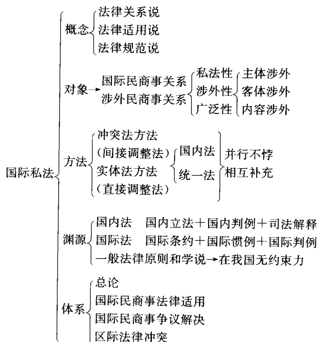
知识逻辑图
