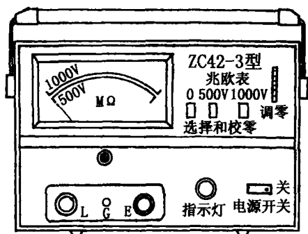
图 1-3 市电式兆欧表外形示意图
