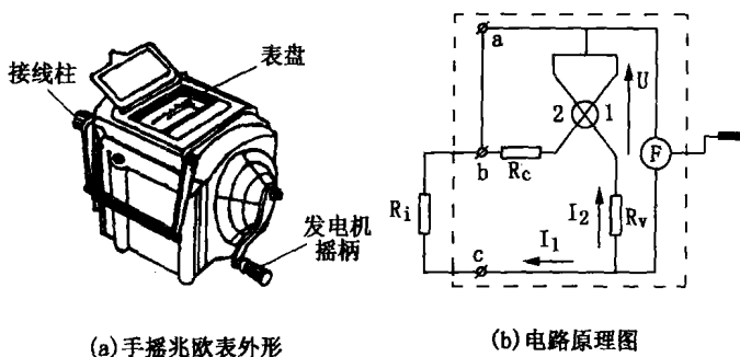
图 1-2 手摇兆欧表外形图和电路图
