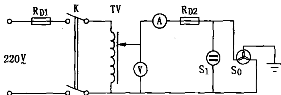
图 1-1 测试配电板电气原理图
