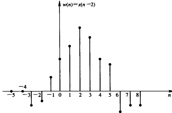
图 1-2 图 1-1 序列 x(n) 的延时
