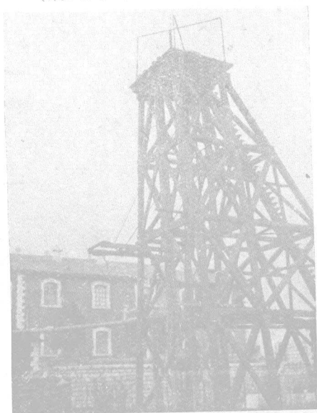
(山礦格拉馬司公務錫) 機降升洞礦式新
