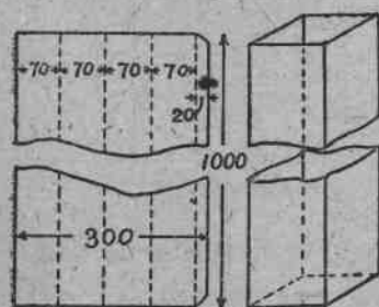
圖14 長方筒
