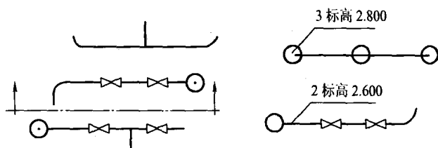
图 1—6 管线的平面图
