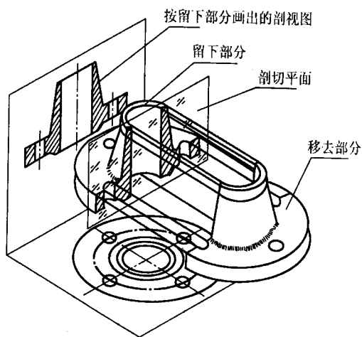
图 1—3 高颈法兰的全剖视图
