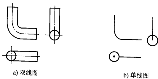
图 1—2 单、双线图
