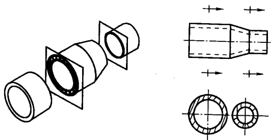
图 1—4 管子的剖视图
