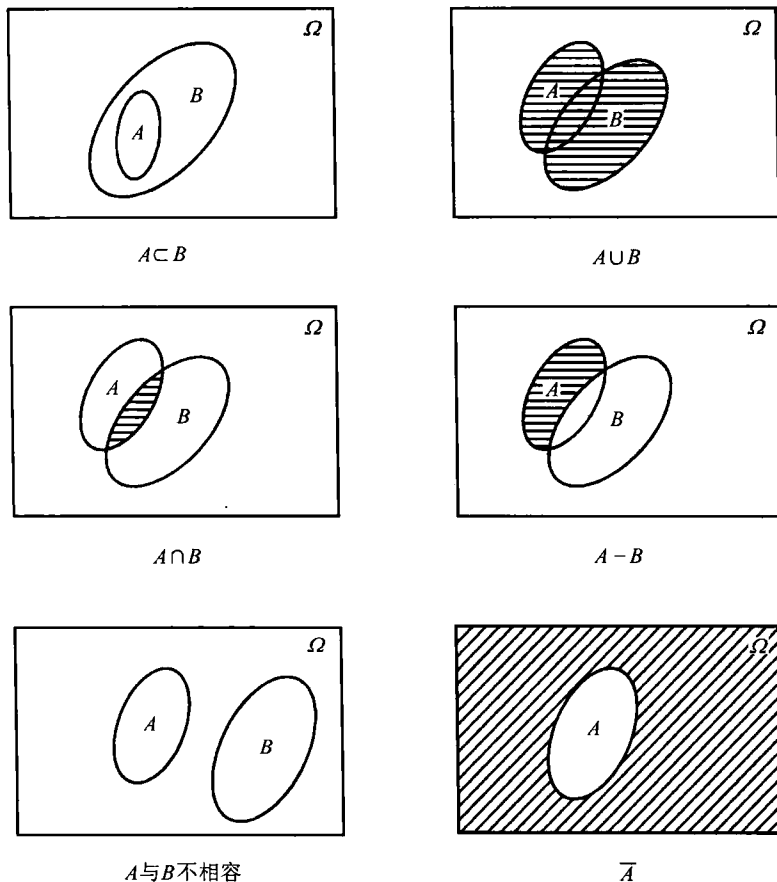
图 1.1 事件的关系与运算的文氏图
