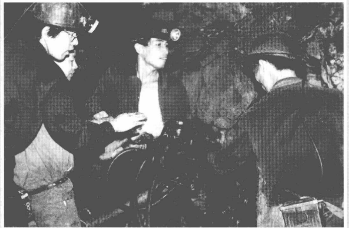
▲ 手持式液压凿岩机在四望嶂矿务局井下作工业性试验。
