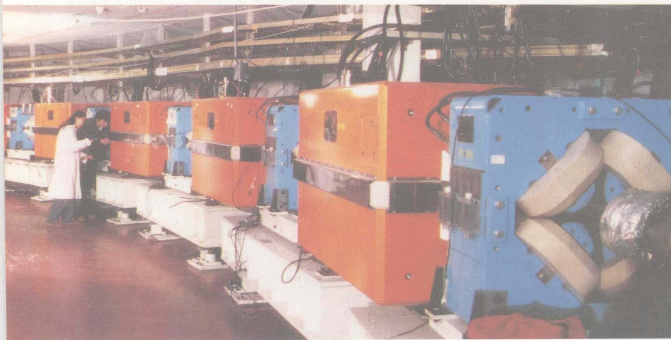
我国建造的第一台高能加速器——北京正负电子对撞机顺利出束
