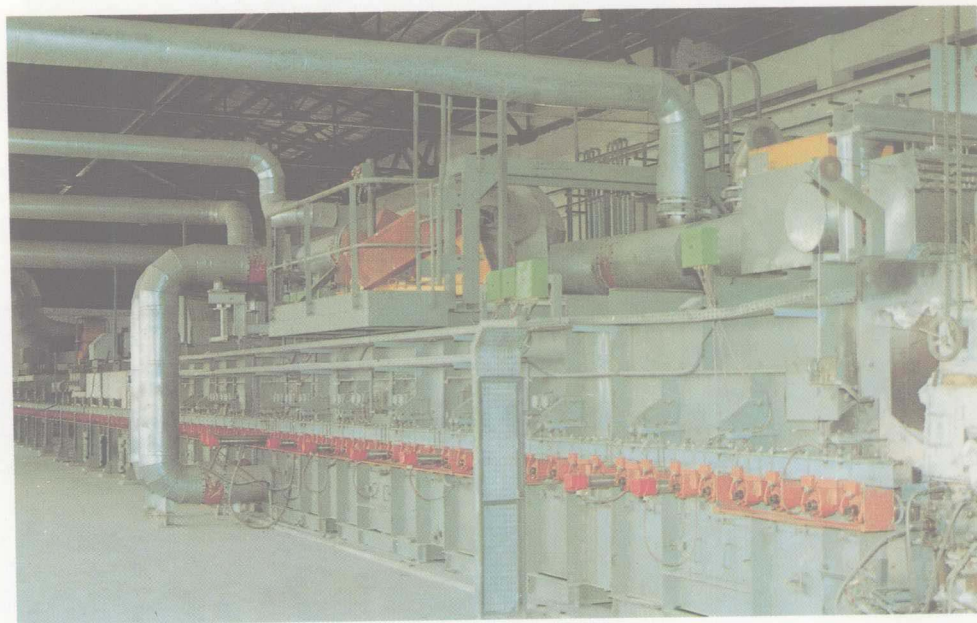
宝钢冷轧厂2030毫米冷连轧机
