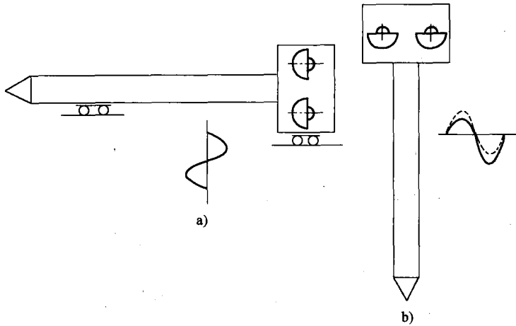
图 2-2 振动桩锤的工作原理
