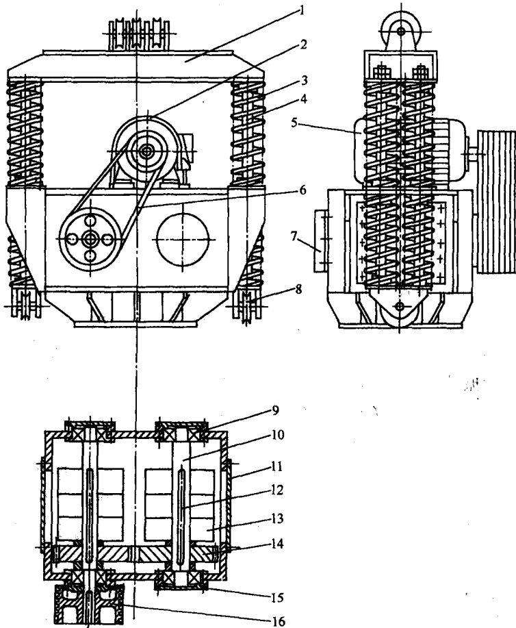
图 2-3 振动桩锤
