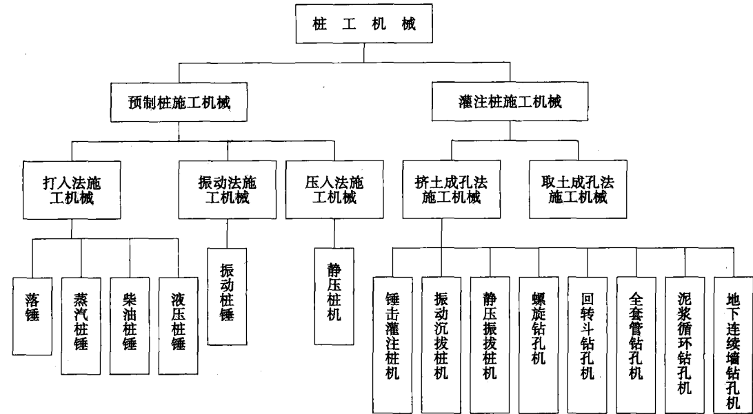
图 1-1 桩工机械分类
