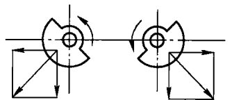
图 2-1 激振力的合成
