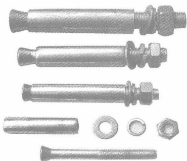
图 1-8 金属膨胀螺栓（普通型）
