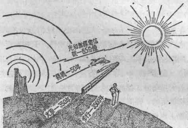
圖2. 太陽離開我們這麼遠
