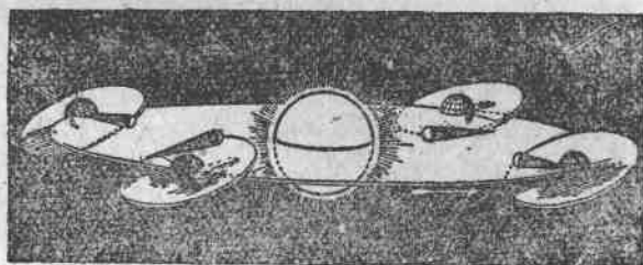
圖 6. 地球和月球繞日運動的情形
