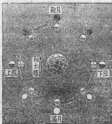
圖 5. 月的位相：在月球軌道外面所畫的便是我們從地球上望見的月的位相
