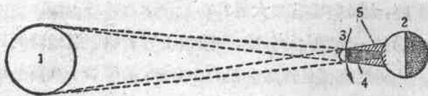
圖 7. 日蝕時地球和月球的位置
