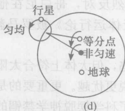
图 1—1 托勒密体系所采用的地心模型
