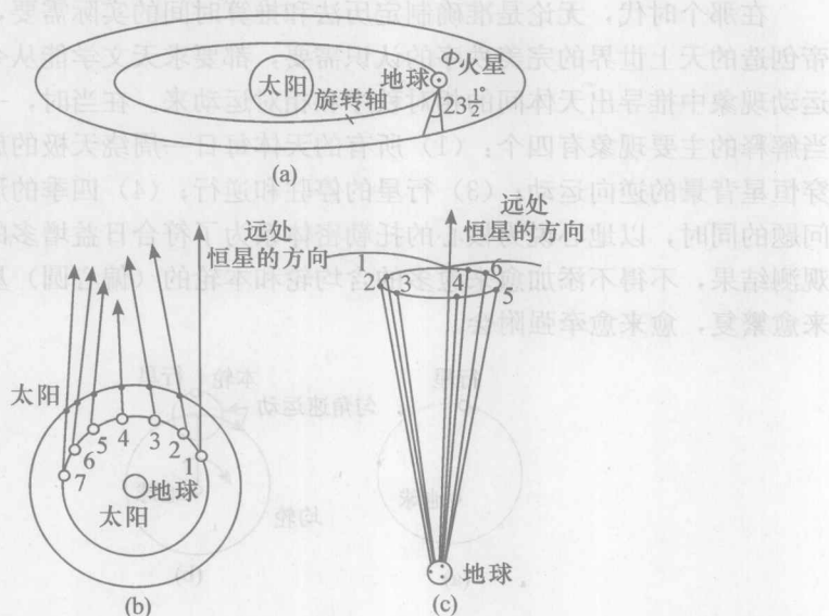
图1—2 哥白尼所采用的日心模型
