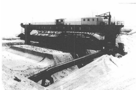
始建于1950年的茶卡盐厂
