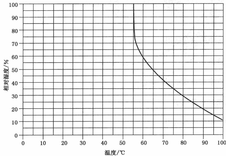
图 102 非正常工作状态下温湿度曲线图
