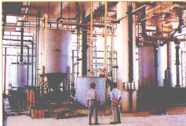
贵州瓮福磷肥厂氟化铝装置
