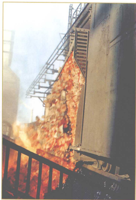
贵阳煤气气源厂（原贵州有机化工总厂焦化分厂1号焦炉投产）
