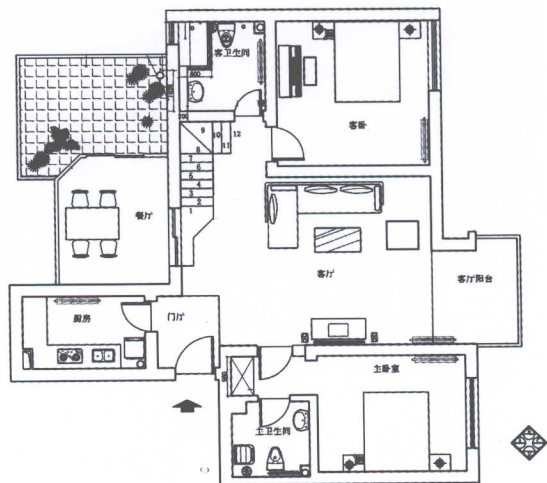
平面布置图
