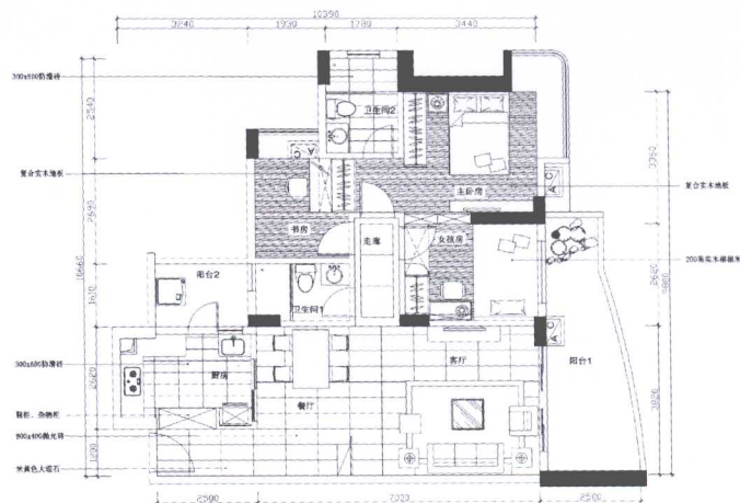
平面布置图
