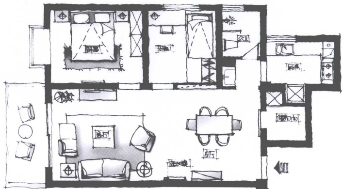
平面布置图
