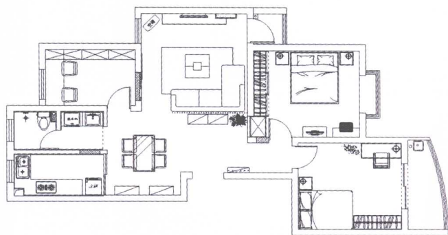
平面布置图
