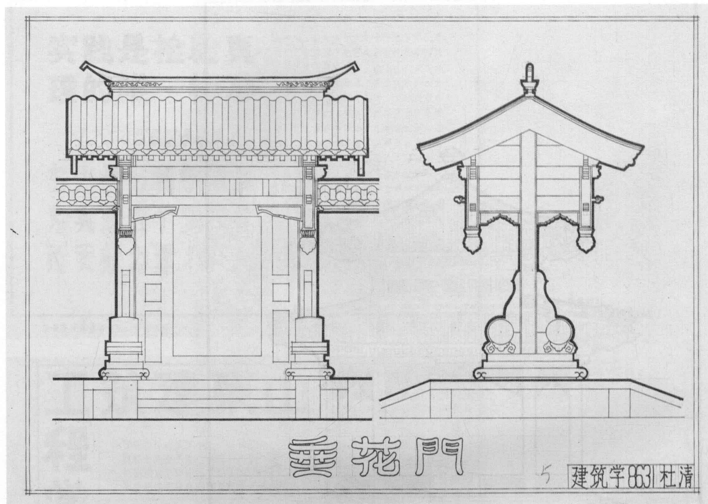
作业名称 垂花门立面抄绘 作者 86 级建筑学 杜清
