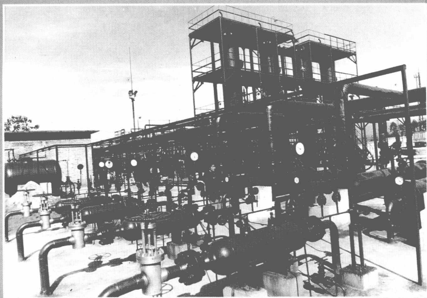
◀ 低温集气站
