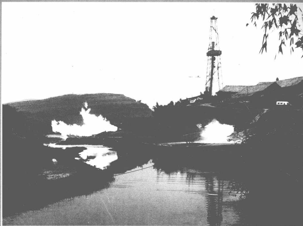
▲ 天然气放喷测试
