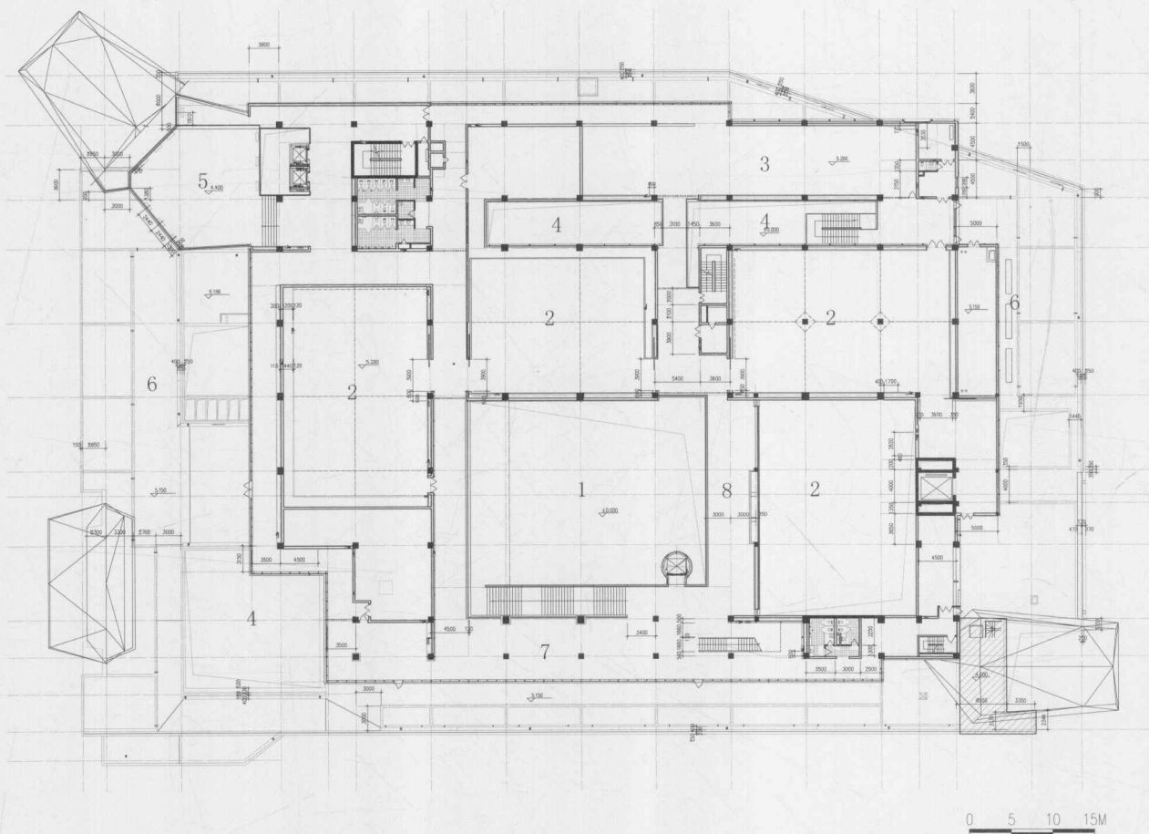
二层平面图 Second Floor Plan
