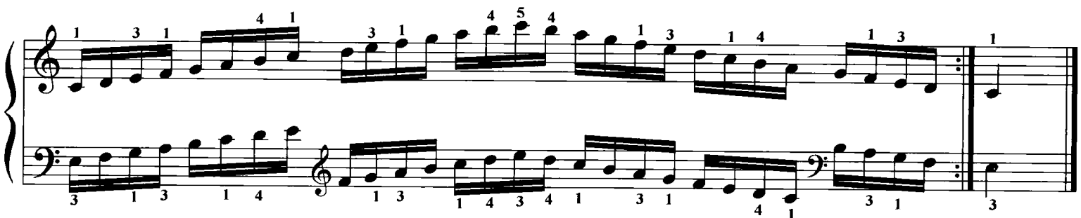
属七和弦
