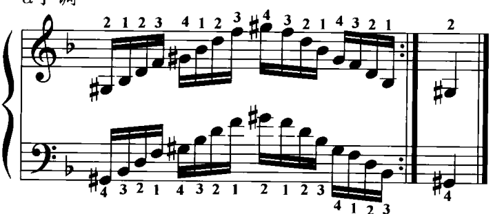
a小调
