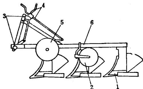
图 1—4 悬挂铧式犁
