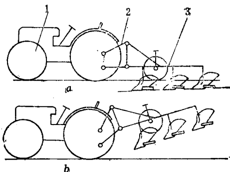
图 1—1 悬挂犁简图
