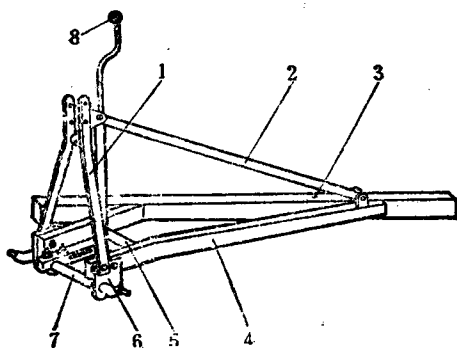
图 1-11 犁架和悬挂装置
