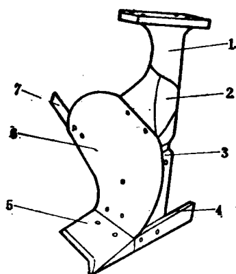
图 1—5 犁体
