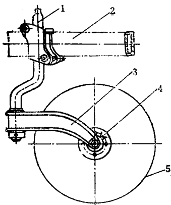
图 1-10 圆犁刀
