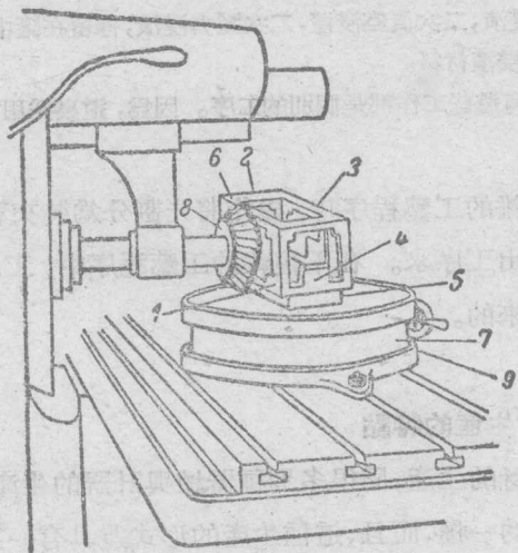
圖1-3 從操作中分析出裝夾和排位的例子。
