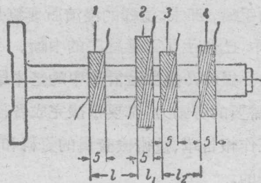
圖 1-2 從操作中分析出四個排位動作的例子：在一個繞圈骨架上纏繞四個萬用線捲。
