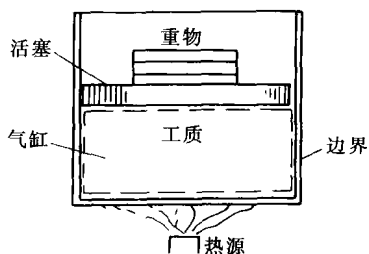
图 1-1 闭口热力系
