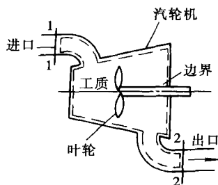
图 1-2 开口热力系
