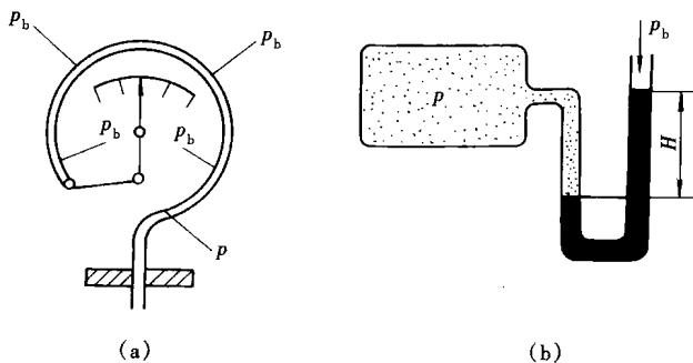
图 1-3 压力的测量
