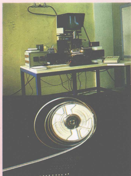
成都无线电四厂从美国引进片状电容生产线车间一角
