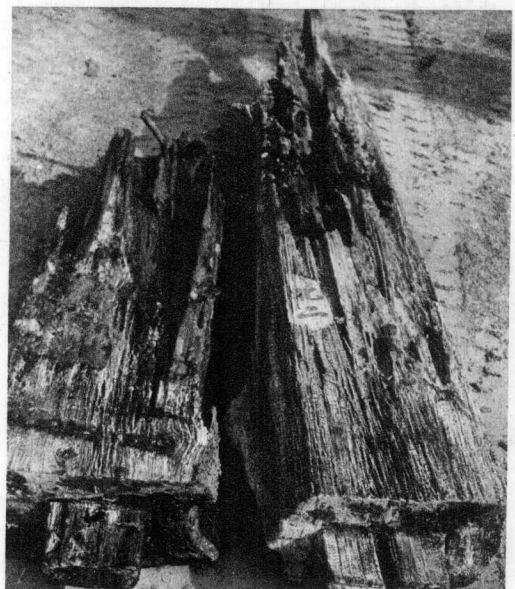
6. 北壁残立木端头的榫
