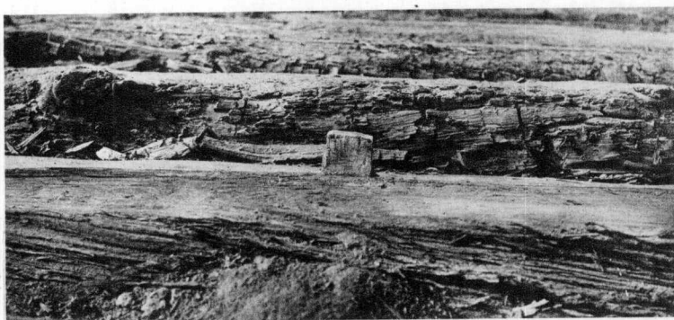
3. 固定棺床木的榫卯
