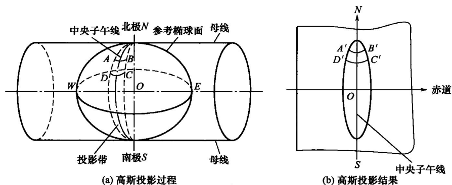
图 1.6 高斯投影
