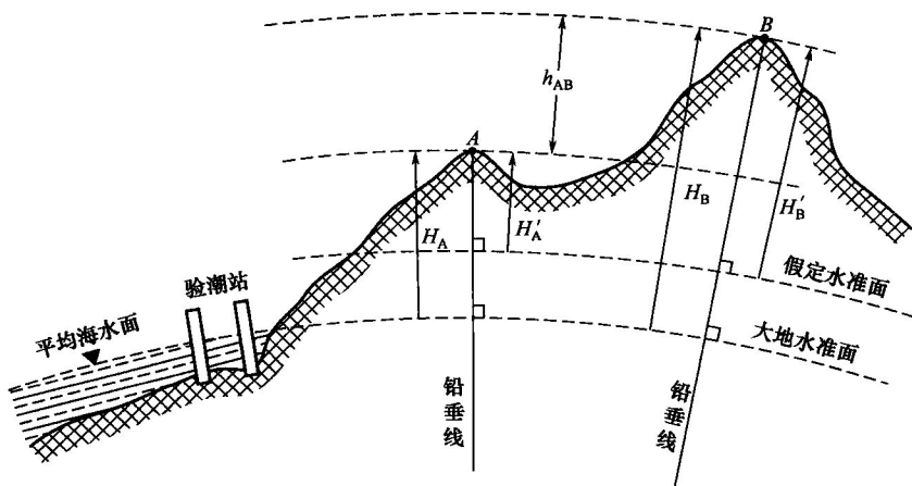
图 1.3 高程和高差
