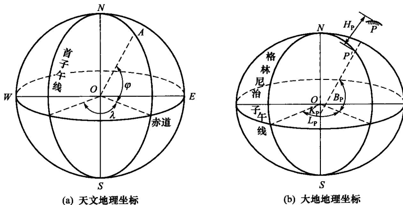
图 1.4 地理坐标示意图
