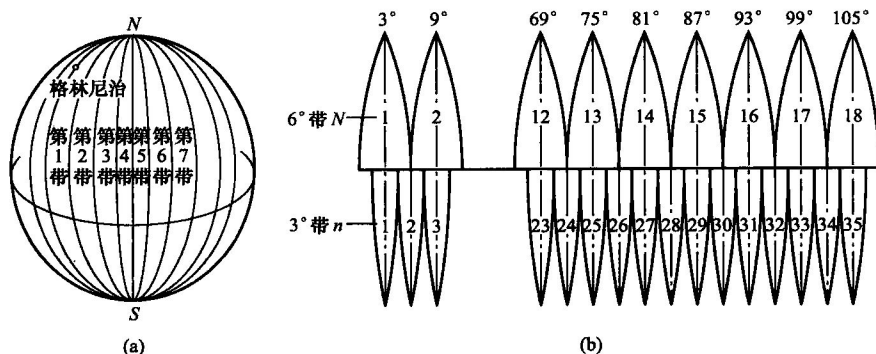
图 1.7 6^\circ 带和 3^\circ 带投影
