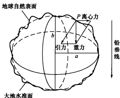
图 1.1 地球重力线
