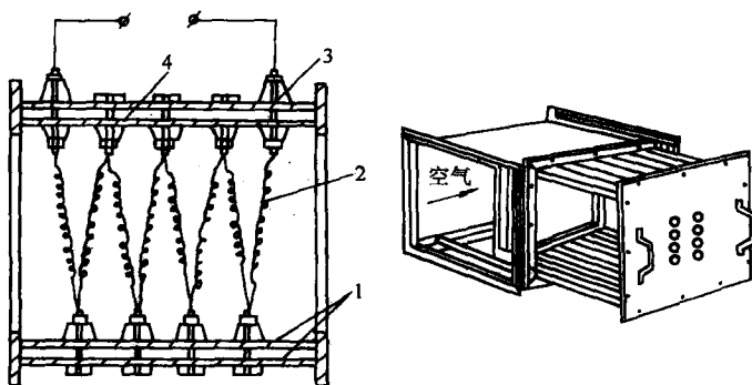
图 1-4 裸线式电加热器
