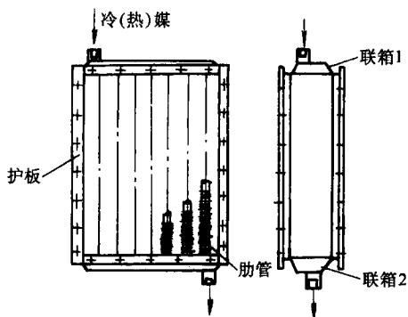
图 1-3 表面式翅片管型空气加热器
