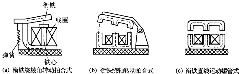
图 1.1 接触器电磁系统的结构图
