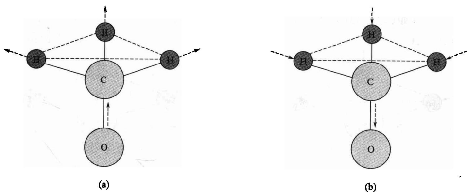
图 1-5 \text{O}-\text{C}-\text{H} 的对称伸缩振动 \nu_s (三个氢原子同时远离或靠向碳原子运动，氧原子与氢原子一样相对于碳原子做相同方向的运动)
