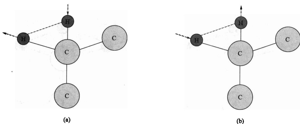
图 1-4 亚甲基 \text{CH}_2 反对称伸缩振动 \nu_s (一个氢原子远离碳原子运动而另一个氢原子靠向碳原子运动)
