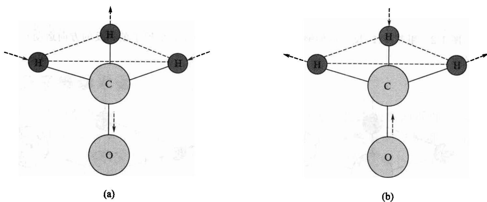
图 1-6 \text{O}-\text{C}-\text{H} 的反对称伸缩振动 \nu_a (一个氢原子远离碳原子而另两个氢原子靠向碳原子运动，或两个氢原子远离碳原子而另一个氢原子靠向碳原子运动)
