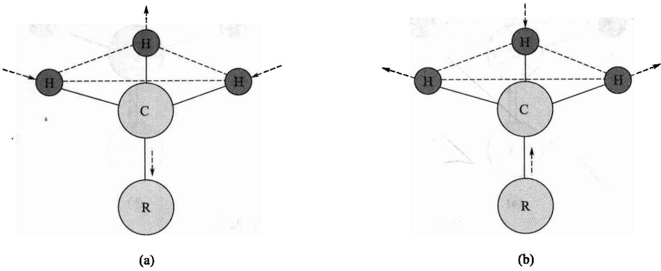
图 1-2 甲基 \text{CH}_3 反对称伸缩振动 \nu_a (相对于碳原子, 氢原子朝相反的方向运动)
