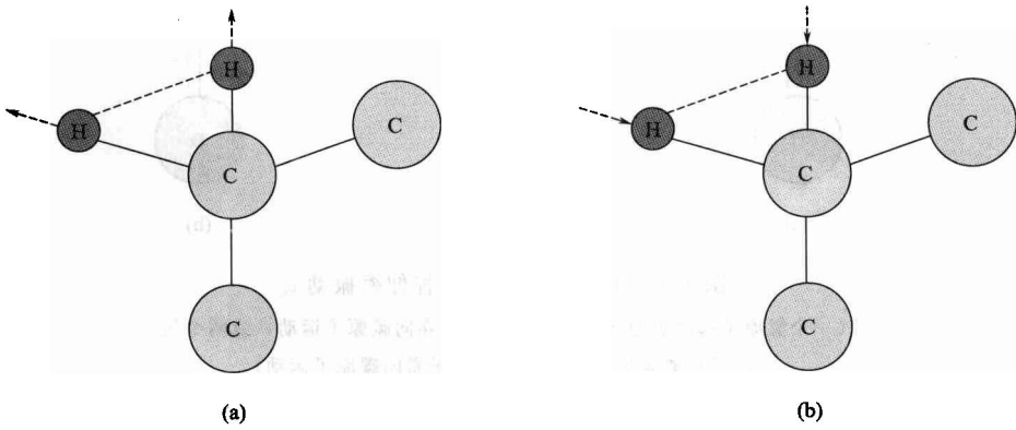
图 1-3 亚甲基 \text{CH}_2 对称伸缩振动 \nu_s (两个氢原子同时远离或靠向碳原子运动)
