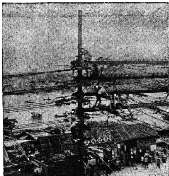
五仙門輸出饋電總牌坊檢修工程，工人同志在積極努力的工作着 ←
