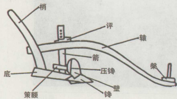
曲辕犁详图
