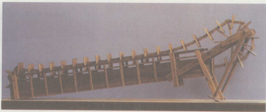
曹魏马钧改进的翻车（复原图）
