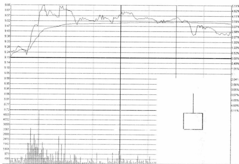
图 1-6 上影阳线
