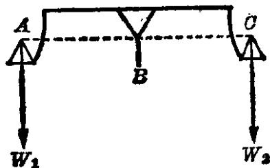
图 1-1 天平构造原理示意图
