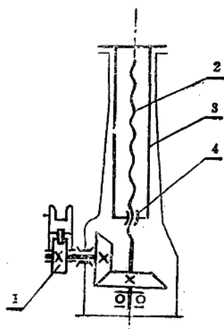
图0-1 螺旋千斤顶
