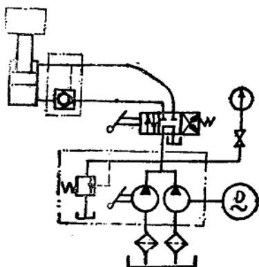
图0-2 FQ系列分离式千斤顶 液压系统图
