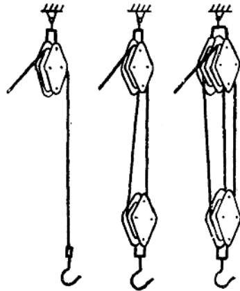
图0—3 不同的定滑车与动滑车
