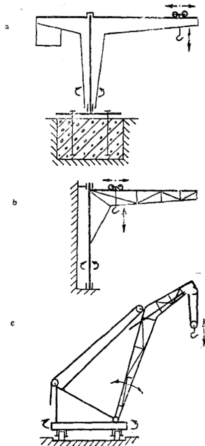
图0—5 固定式旋转起重机
