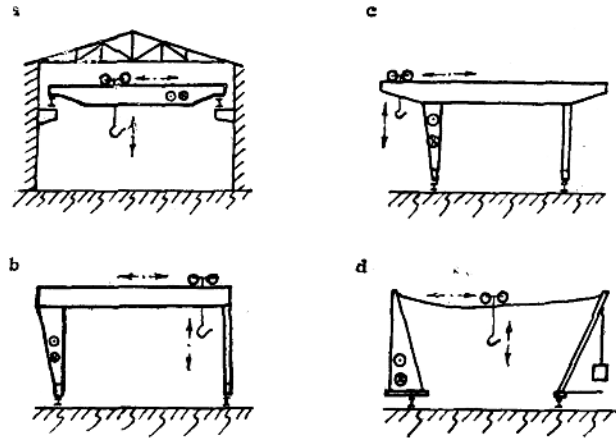
图0—4 桥式类型起重机主要型式
