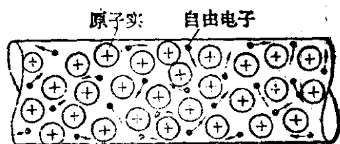
图 1-1 金属中的原子实和自由电子
