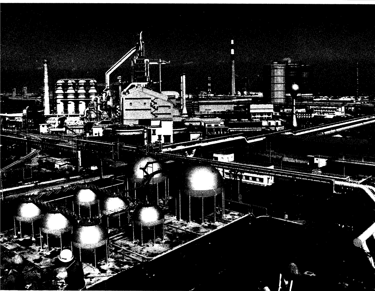
中国现代化的大型钢铁企业——宝山钢铁总厂一角
