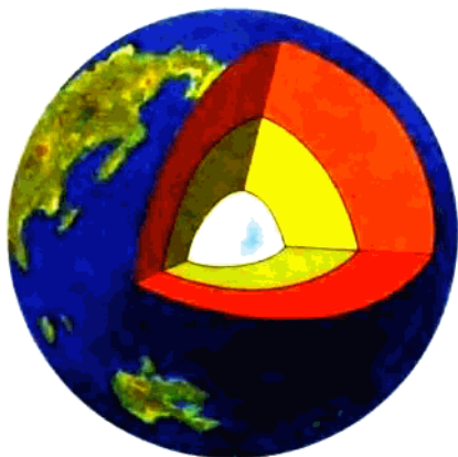
地球的构造
