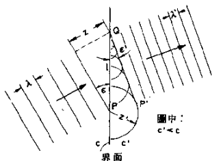
圖 1.3 Huygens 單元波折射情形
