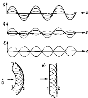
圖 1.2 波的干涉。a, b, c 表示兩個波間的干涉；d, e 表以 Huygens 單元波造成球波擴展和平波擴展。
