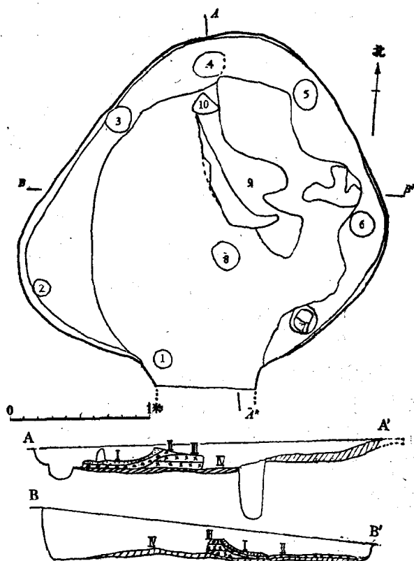
图六 F3平、剖面图 (1/40)
