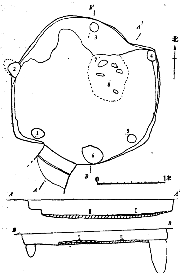
图五 F2平、剖面图 (1/40)
