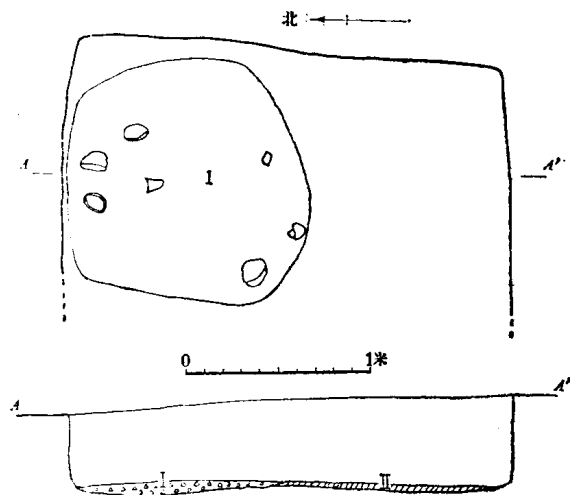
图八 F1平、剖面图 (1/40)
