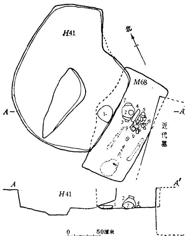
图四 H41、M68平、剖面图
