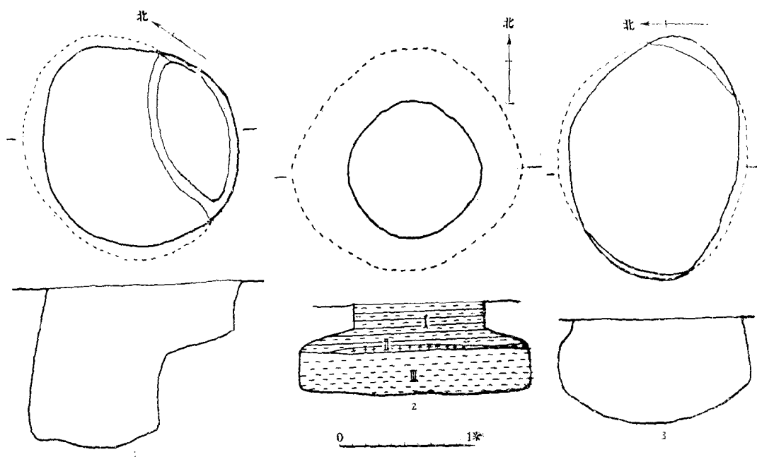
图九 灰坑平、剖面图
