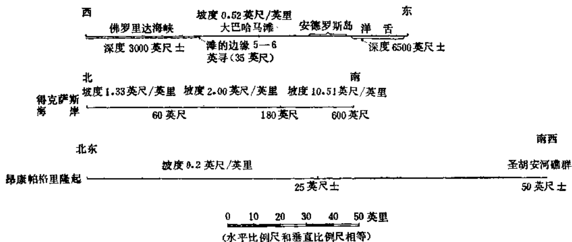
图 2 现代海底及陆表海海底的坡度
