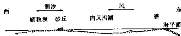
图 3 朱尔特礁岛区的环境模式
