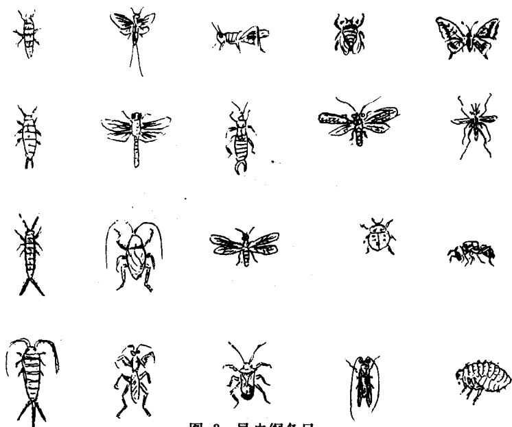
图 3 昆虫纲各目
