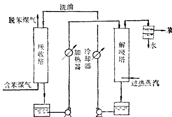
图 8-1 吸收与解吸流程
