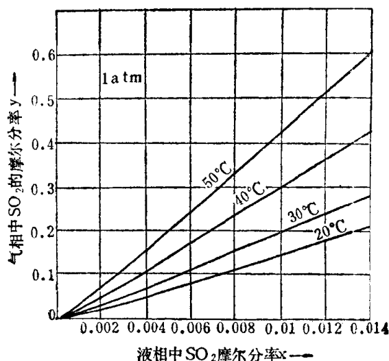
图 8-4 1atm下SO 2 在水中的溶解度
