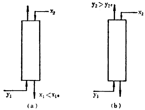
图 8-7 吸收过程的极限
