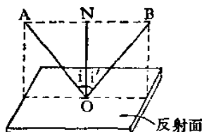
光の反射
